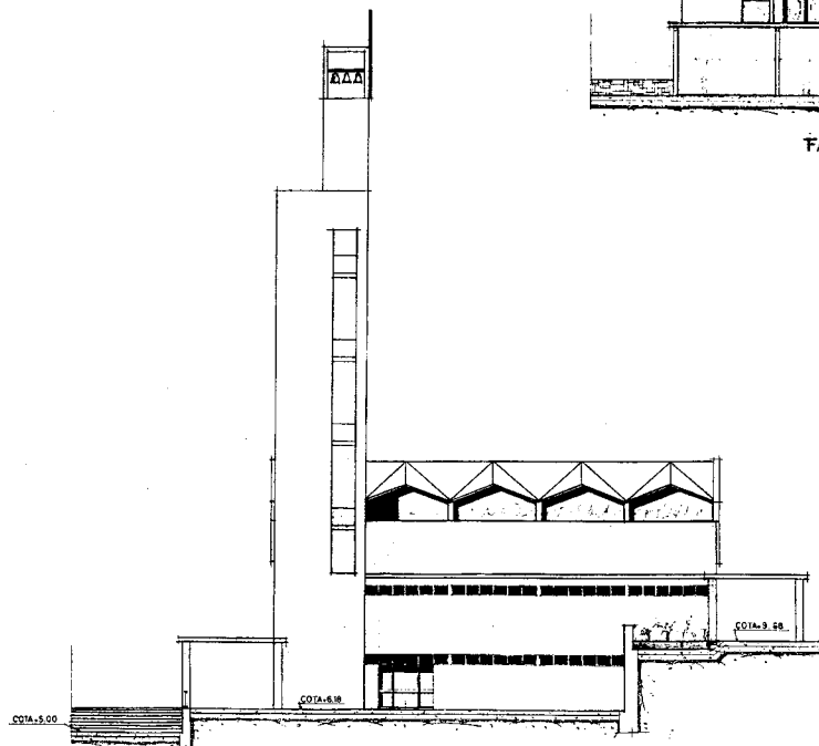
FACHADA LATERAL IZQUIERDA
